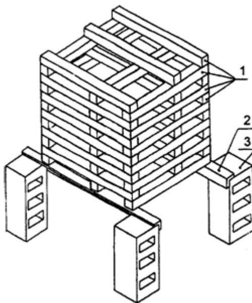
1 - деревянные бруски; 2 - стальной уголок; 3 - бетонный (металлический) блок
